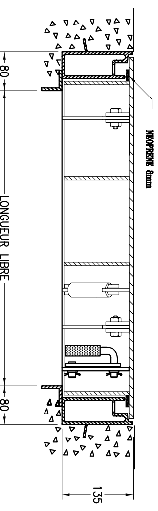
COUPE B-B
