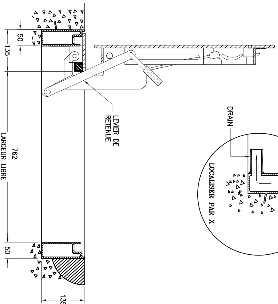
COUPE A-A ECH. P.A.E.
