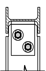
COUPE C-C
