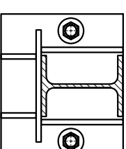
COUPE A-A ARRANGEMENT TYPIQUE
